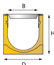
zamocowanie zatrzaskowe
